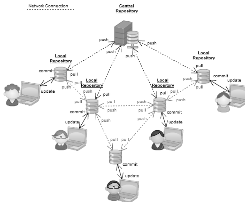
Fig. 2: Visar upplägget i ett decentraliserat versionshanteringsystem. Alla användare kan koppla upp sig mot ett centralt repo men kan också dela filer mellan varandra
