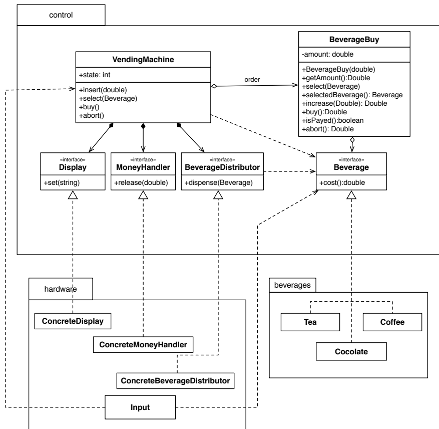
Figur 1: Klassdiagram kaffeautomat
