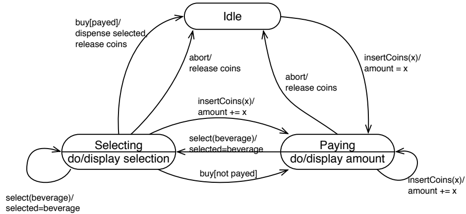
Figur 2: Tillståndsdigram kaffeautomat
