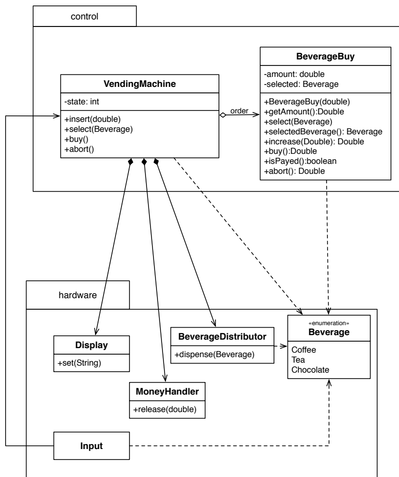
Figur 1: Klassdiagram kaffeautomat
